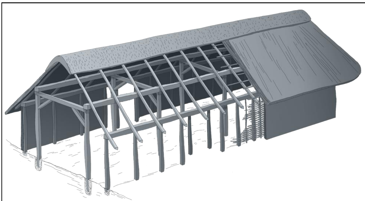
Fig. 7: Rekonstruktionstegning af et treskibet langhus med sætvis tagbærende stolper og vægstolpehuller. Illustration: Jeanette Nørgaard, © Viborg Museum
